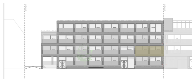
Voorraanzicht
